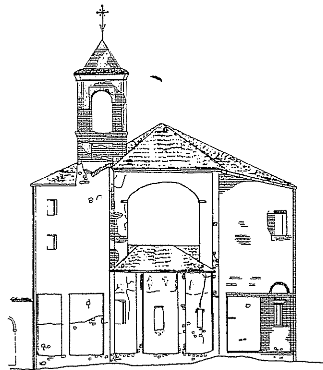
PROSPETTO EST
